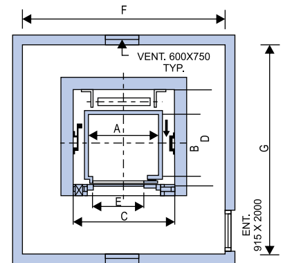
HOIST WAY PLAN FOR MANUAL DOOR
