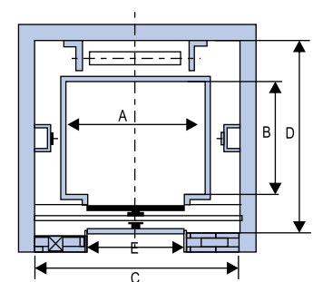
HOIST WAY PLAN FOR AUTO DOOR
